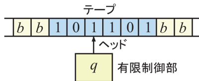
図 4・2 チューリング機械の概念図
